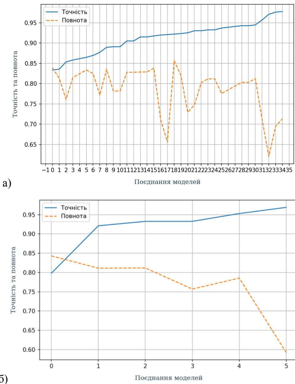
Рис. 7.7. Макрохарактеристика точності та повноти поєднань рішень СПР (клас 5): а – поєднань рішень СПР: б – СПР ансамблю
