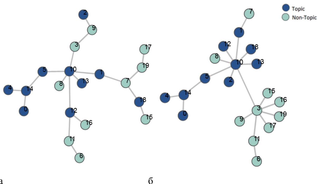
Рис. 7.8. МОД нетипових даних (клас 1): а – множина ознак нетипових даних початкова; б – множина нетипових даних із зміненими ознаками <438, 616, 690>, спільними для даних класу і даних поза межами класу
