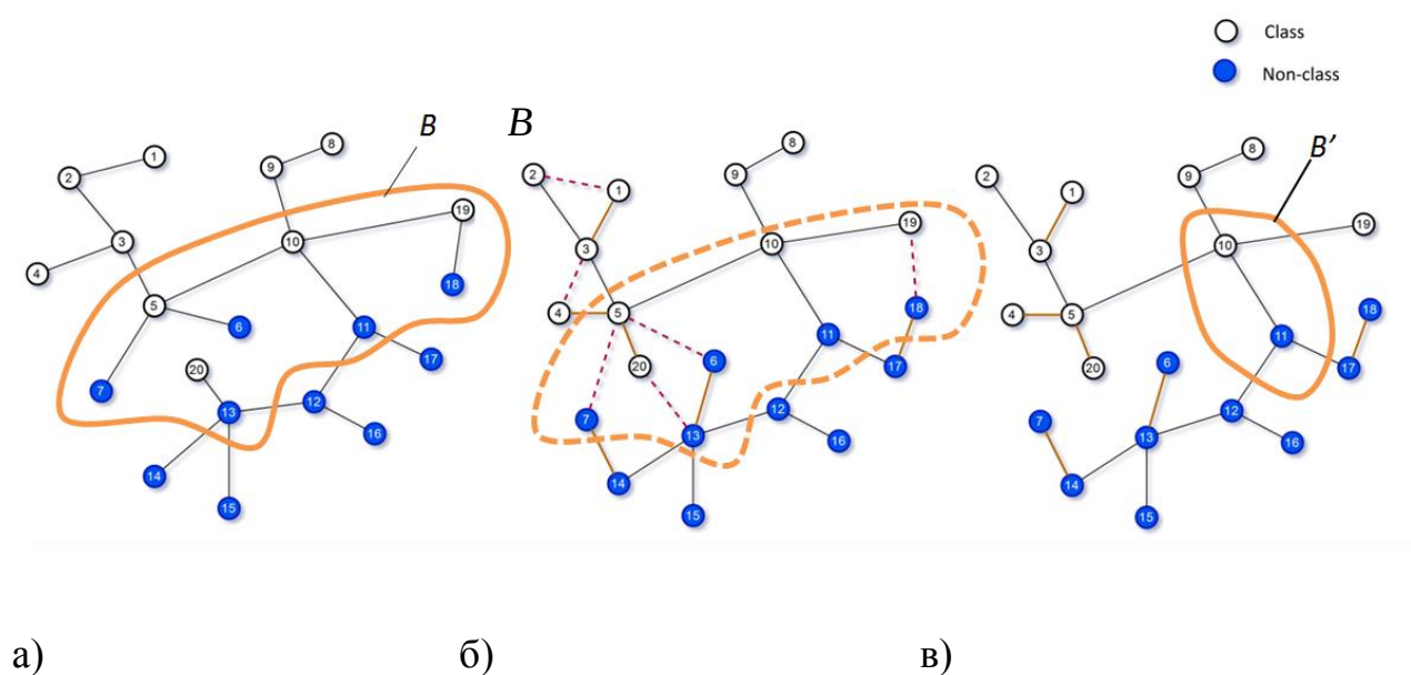
Рис. 5.8. Ілюстрація етапів просторового зміщення з трансформацією МОД зони нетипових даних з виділенням двочасткового субграфа та його мінімізацією (у найкращому випадку двочастковий граф має мінімально можливе значення кількості ребер, яке дорівнює 1). B – початковий двочастковий субграф МОД, B' – двочастковий субграф МОД після просторового зміщення вершин МОД. Штриховою лінією позначені ребра МОД, які зникають після трансформації дерева: а) початкове МОД з двочастковим субграфом; б) трансформація МОД; в) просторово-трансформоване МОД з двочастковим субграфом
