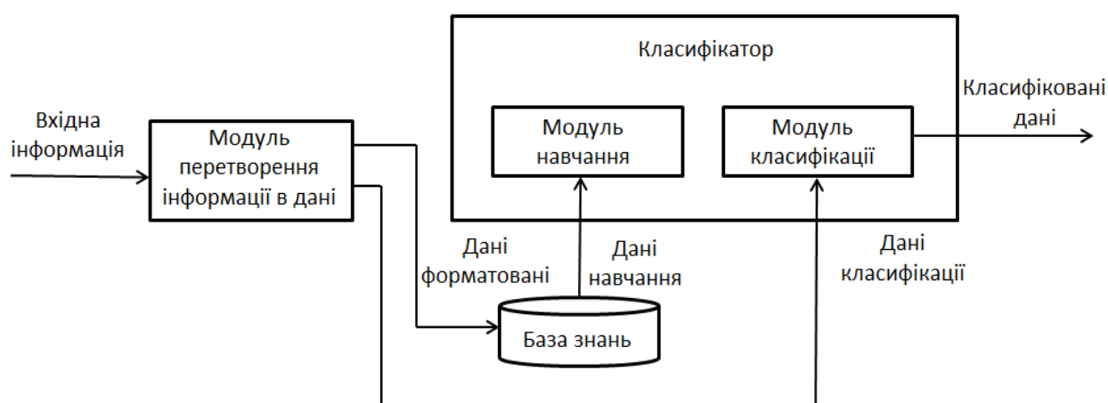
Рис. 3.2. Структура системи прийняття рішення
