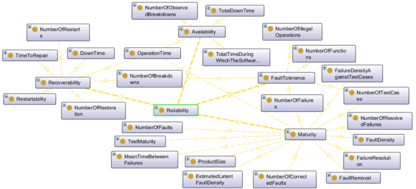
Рис 2.6 – Базова онтологія для Надійності [1]
