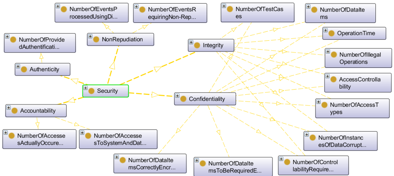
Рис. 2.7 – Базова онтологія для Захищеності [1]
