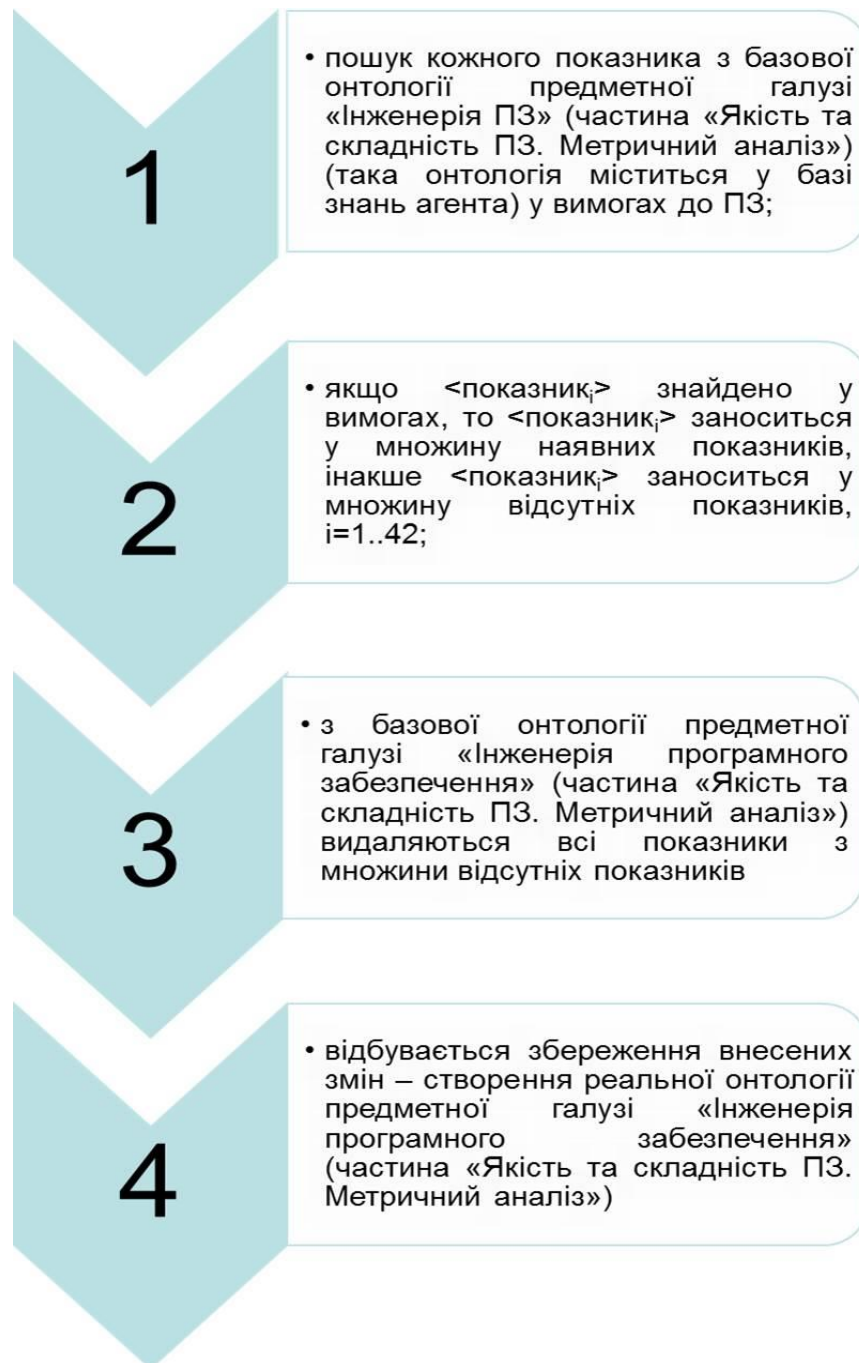
Рис. 3.2 – Метод діяльності інтелектуального агента для семантичного аналізу програмних вимог для пошуку показників для метричного аналізу
